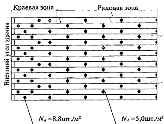
Пример фрагмента теплоизоляции стен до отм. +16,0 от уровня отмостки здания
