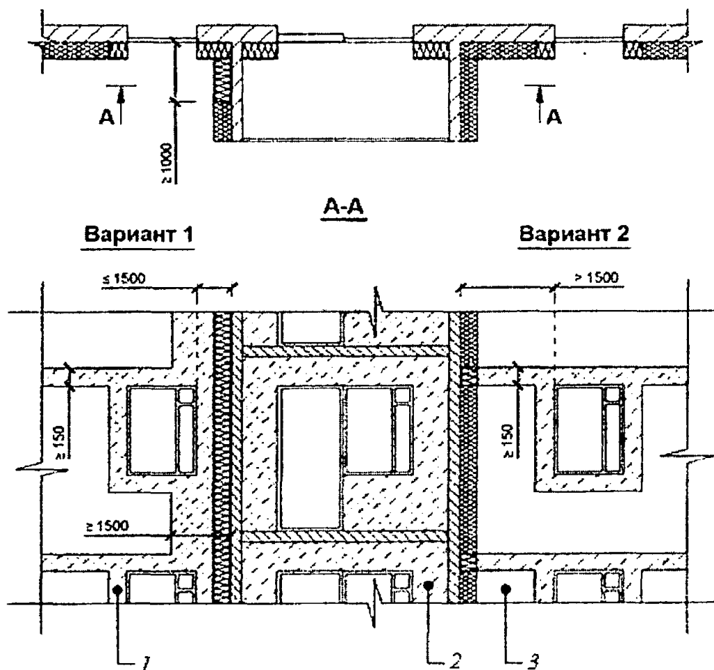
1 - рассечка из изделий из негорючей (НГ) MW; 2 - изделия из негорючей (НГ) MW; 3 - плита из EPS или XPS
