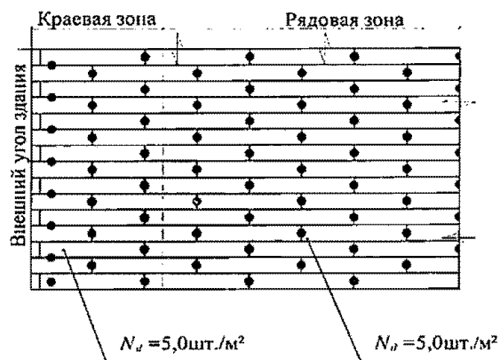
Пример фрагмента теплоизоляции стен до отм. +16,0 от уровня отмостки здания
