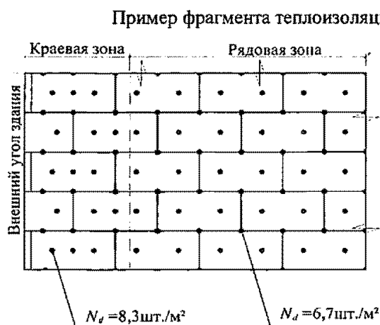
Пример фрагмента теплоизоляции стен до отм. +40,0 от уровня отмостки здания
