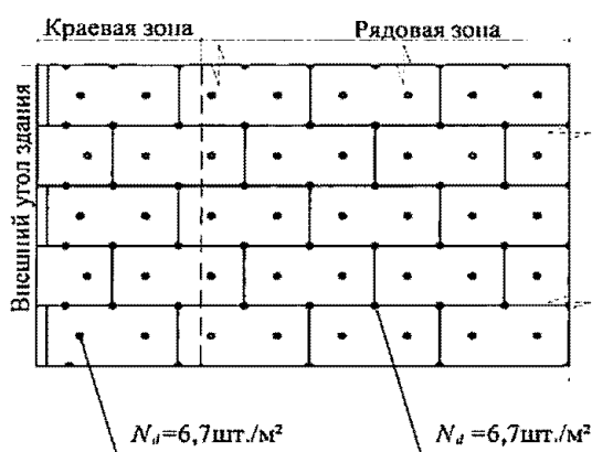
Пример фрагмента теплоизоляции стен до отм. +16,0 от уровня отмостки здания
