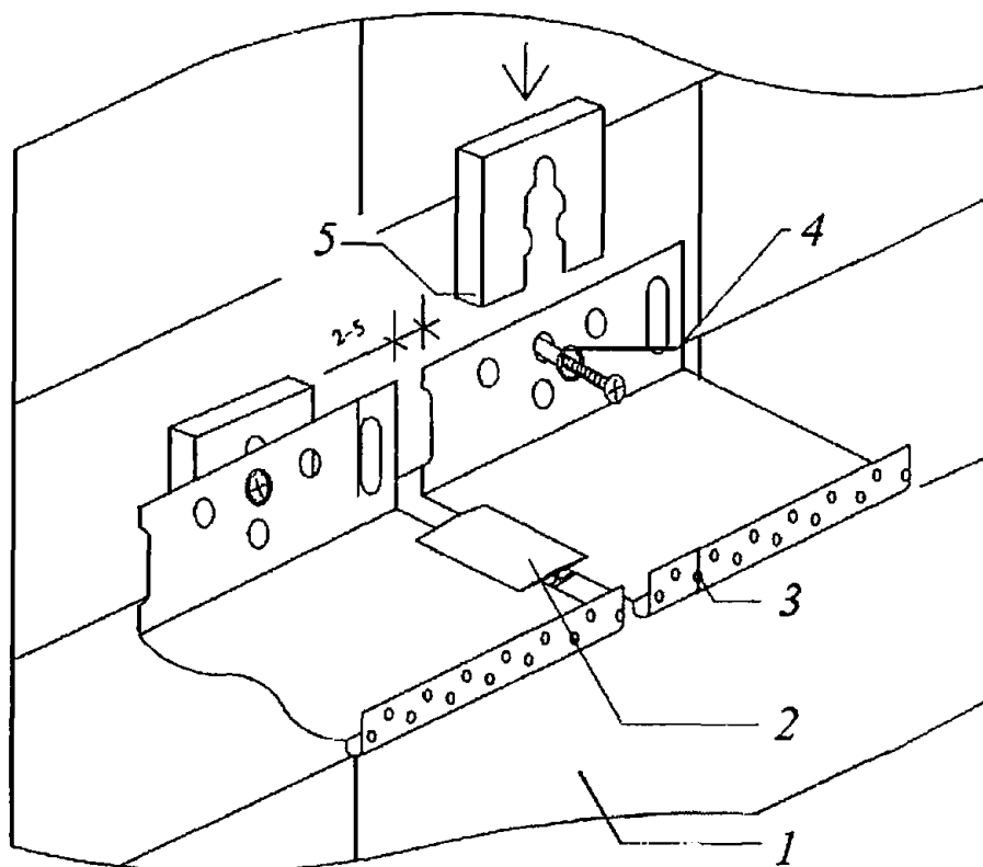
1 - строительное основание; 2 - соединительный элемент цокольного профильного элемента; 3 - опорный цокольный профильный элемент; 4 - анкер с дюбелем; 5 - дистанционная прокладка
